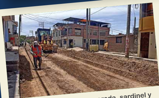
Renovación de berma, vereda, sardinel y calzada en la Calle Tupac Amaru cuadras I,II,III.
